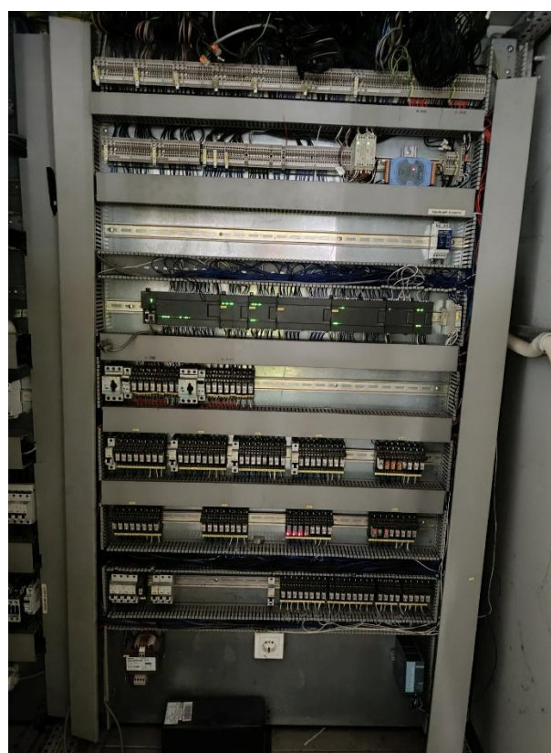
PLC vezérlő rész
